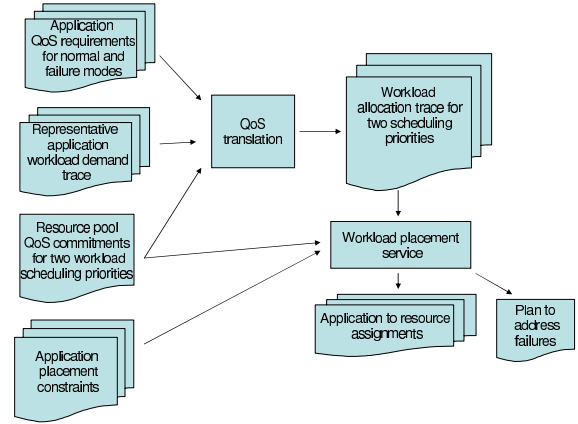
Fig. 2. R-Opus.
